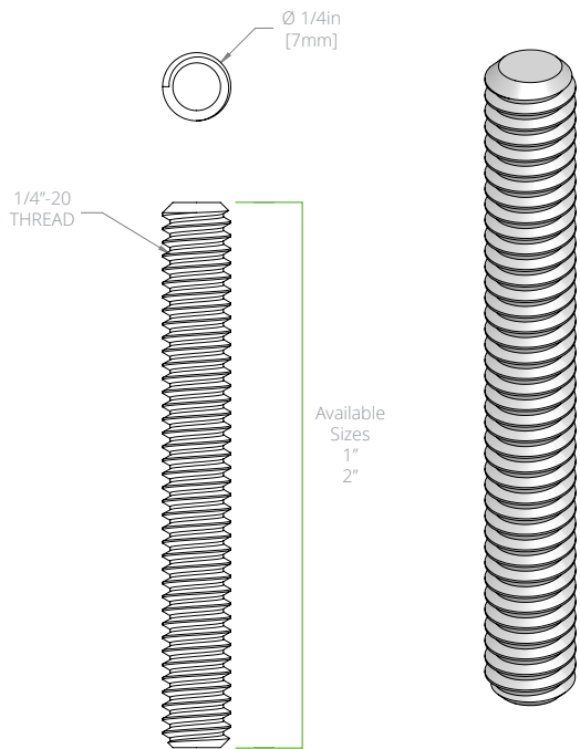
1/4"-20 STUD
