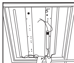
4 Connecter la ligne d'entrée et la ligne de sortie du pilote.
