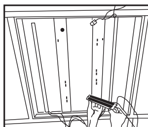
3 Installer le pilote DEL à l'aide du support magnétique.
