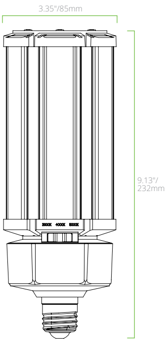
45W & 54W - E26 HIGH VOLTAGE
