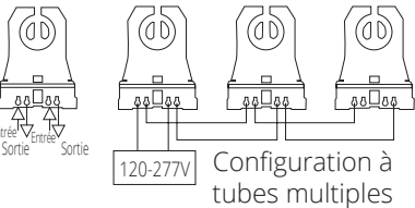
Douilles-supports non shuntées (douilles)
