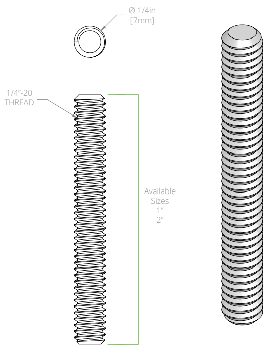
1/4\"-20 STUD
