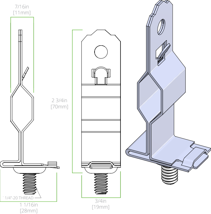
T-BAR W/ 1/4"-20 STUD
